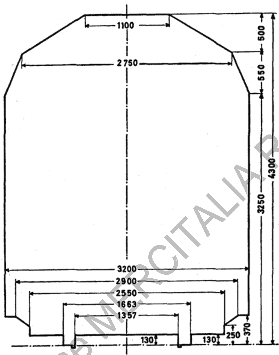
8.7 Tavola 1 7 : Profilo Limite di carico ammesso da RFI (FS), FN
