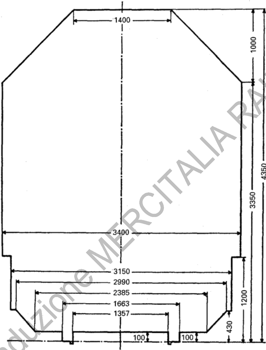
8.15 Tavola 1 15 : Profilo limite di carico ammesso da C (NSB)
