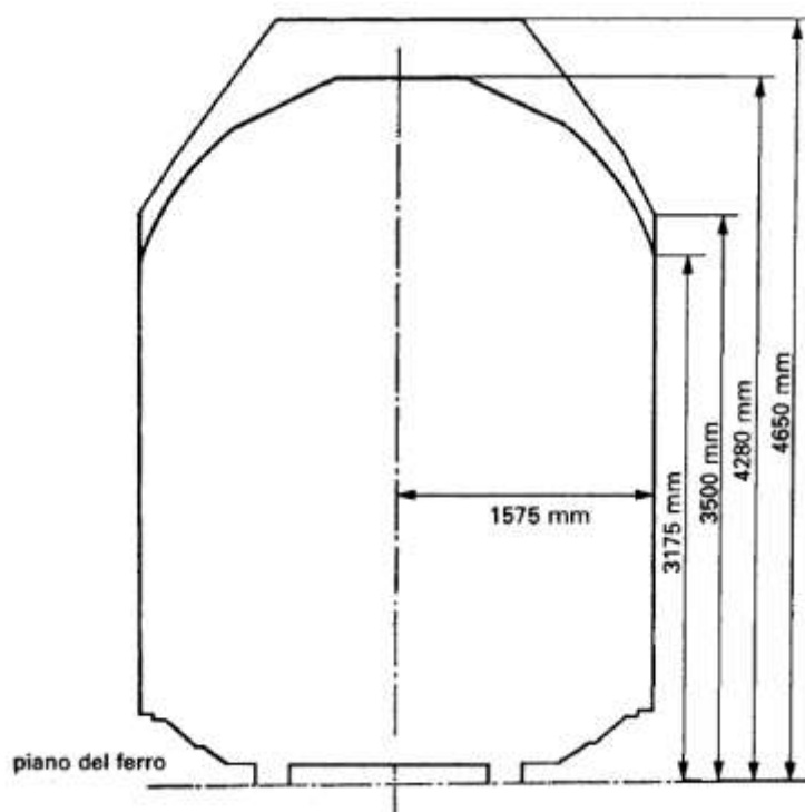
Profilo limite di carico
